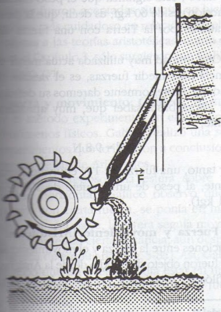
FIGURA 5-3 El chorro de agua ejerce una fuerza sobre las paletas de la turbina.
